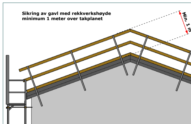
Sikring av gavl med rekkverkhøyde 1 m over takplanet.
